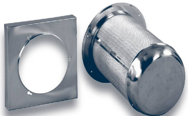
Fästplatta för montering mot kanal och metallfilter med uppsamlings-skål.
